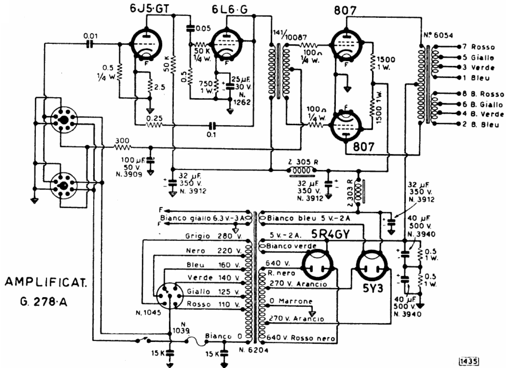
Lo schema elettrico dell'unità di potenza G. 278/A.
